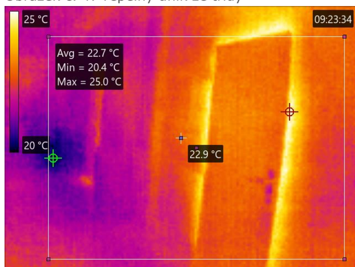
Obrázek č. 4: Tepelný únik ze třídy
